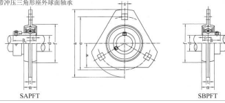
带冲压三角形座外球面轴承
