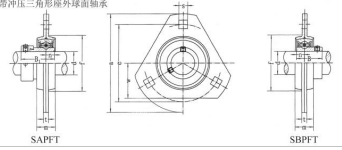
带冲压三角形座外球面轴承
