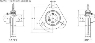
带冲压三角形座外球面轴承
