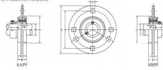
带冲压圆筒形外球面轴承
