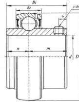
UCX00 (medium-duty)
